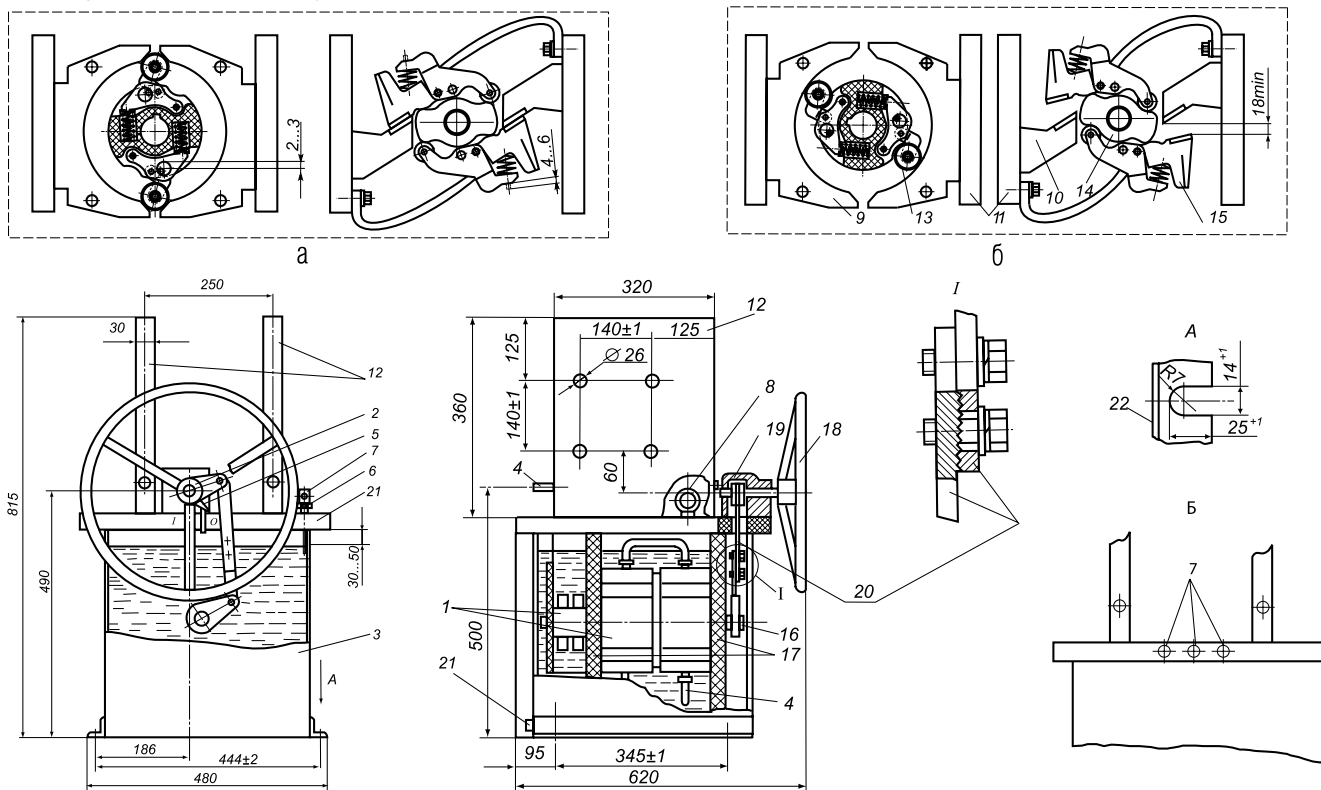
Рисунок 1 Габаритные и установочные размеры выключателя
